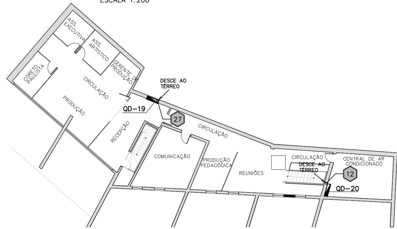
PLANTA BAIXA – TEATRO 2º PAV. – ESCRITÓRIOS ESCALA 1:200
