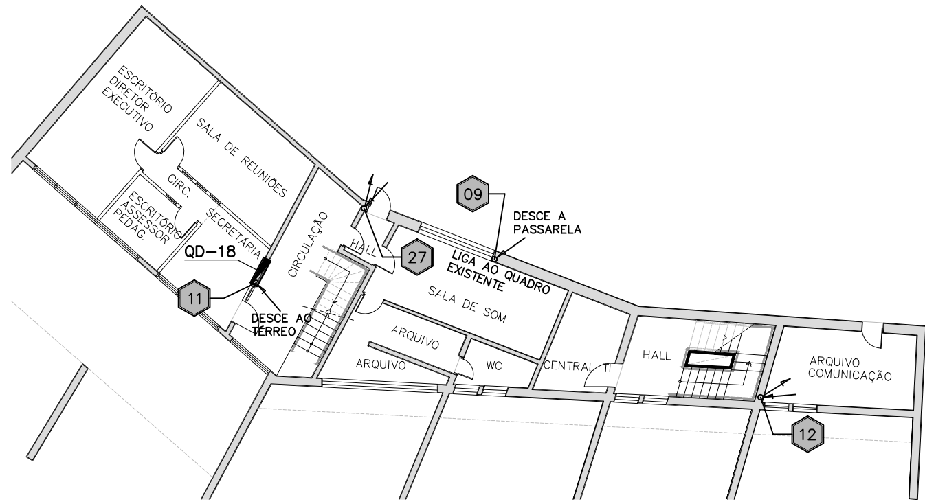
PLANTA BAIXA – TEATRO 1º PAV. – ESCRITÓRIOS ESCALA: 1:200
