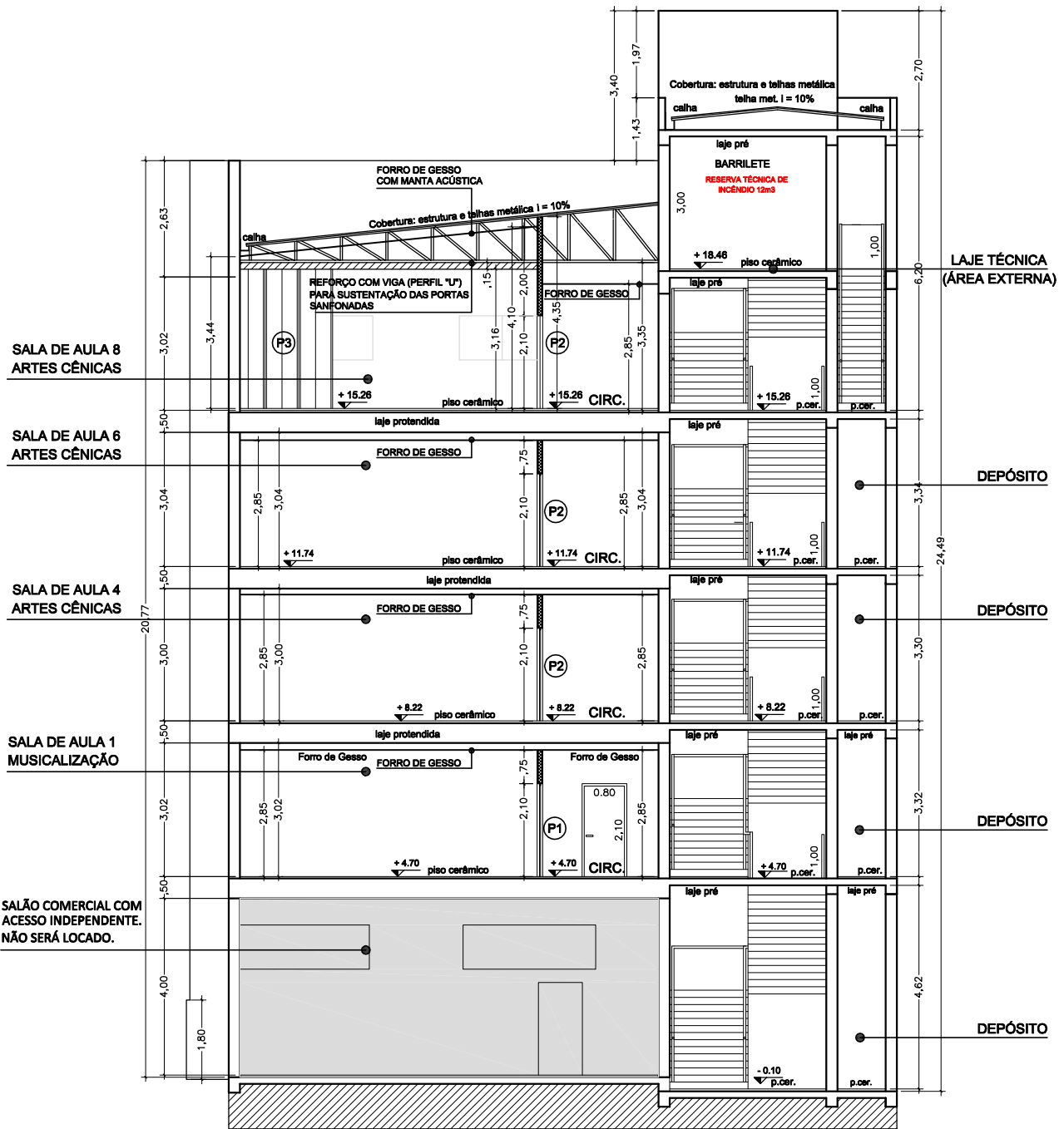
A CORTE AA s/esc
